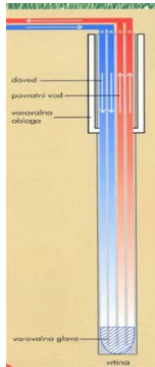
shema sonde
